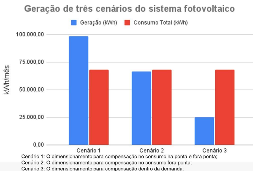
Figura 2 - Geração de três cenários do SF.
