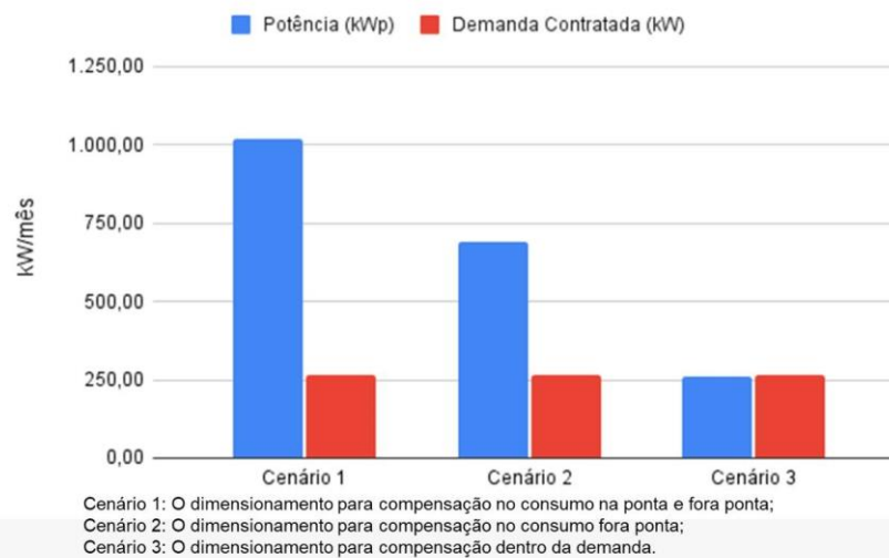
Figura 3 - Relação da potência do SF com a demanda contratada.
