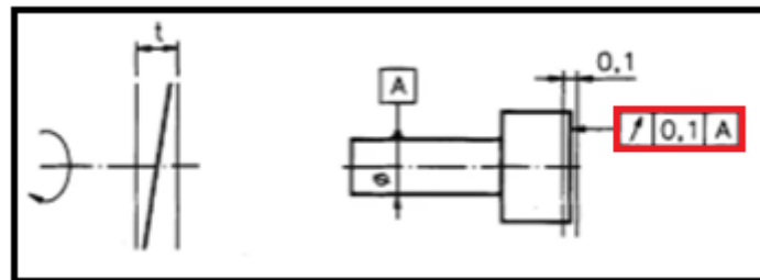
Figura 3 – Medição de batimento axial
