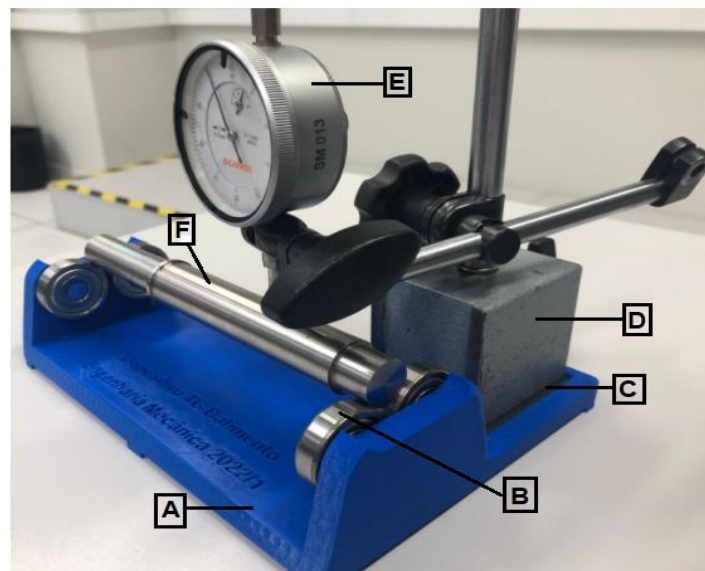
Figura 8- Dispositivo didático para análise de batimento
