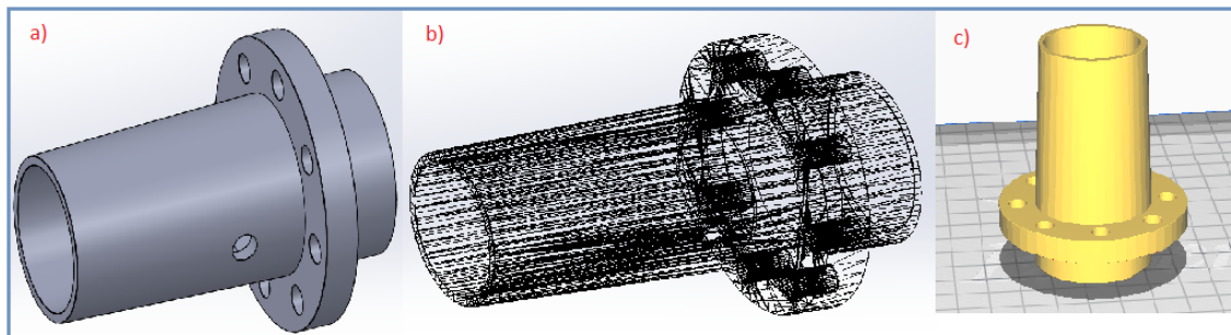
Figura 1 – Transformação da peça CAD para impressão 3D
