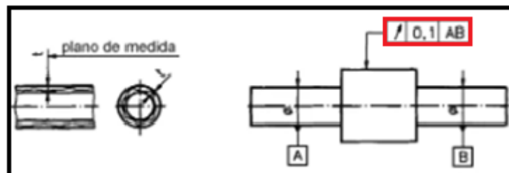
Figura 4 - Medição de batimento radial
