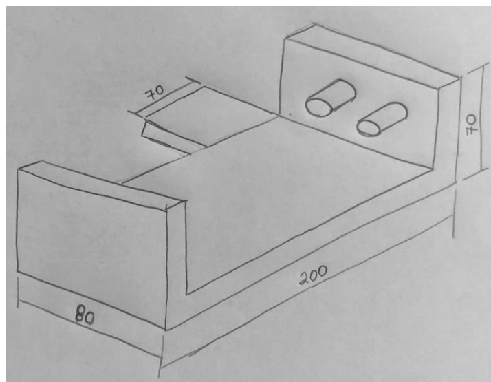
Figura 6 - Esboço inicial
