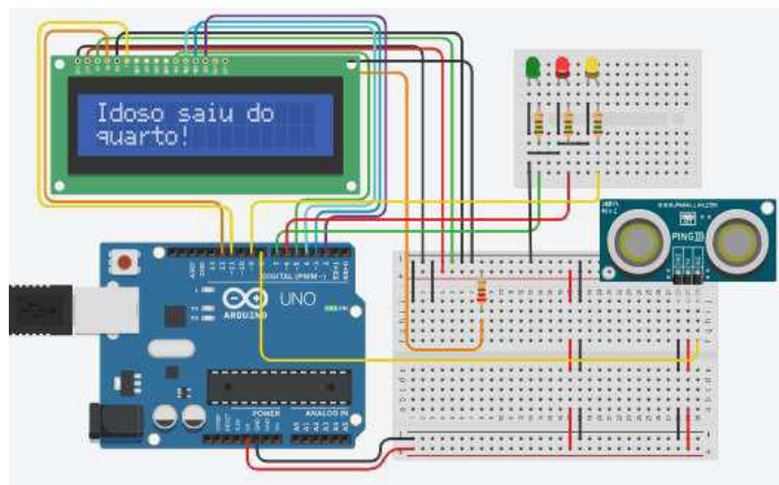
Figura 1 – O circuito esquematizado na plataforma virtual.
