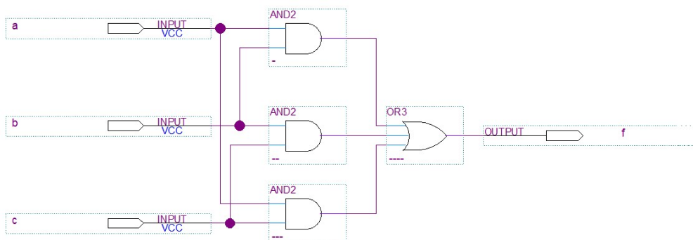
Figura 5 – Design do circuito f = ab + bc + ac
