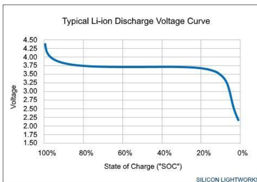
Figura 1 – Típica curva de descarga das baterias de L-ion.
