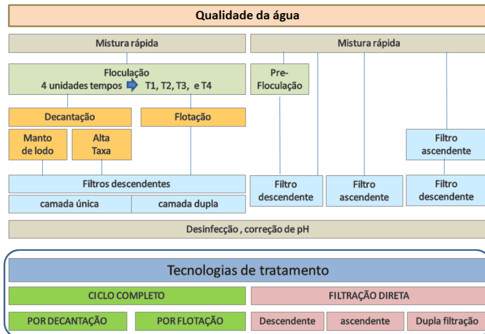
Figura 1 - Esquema descritivo das tecnologias de tratamento de água da IP.
