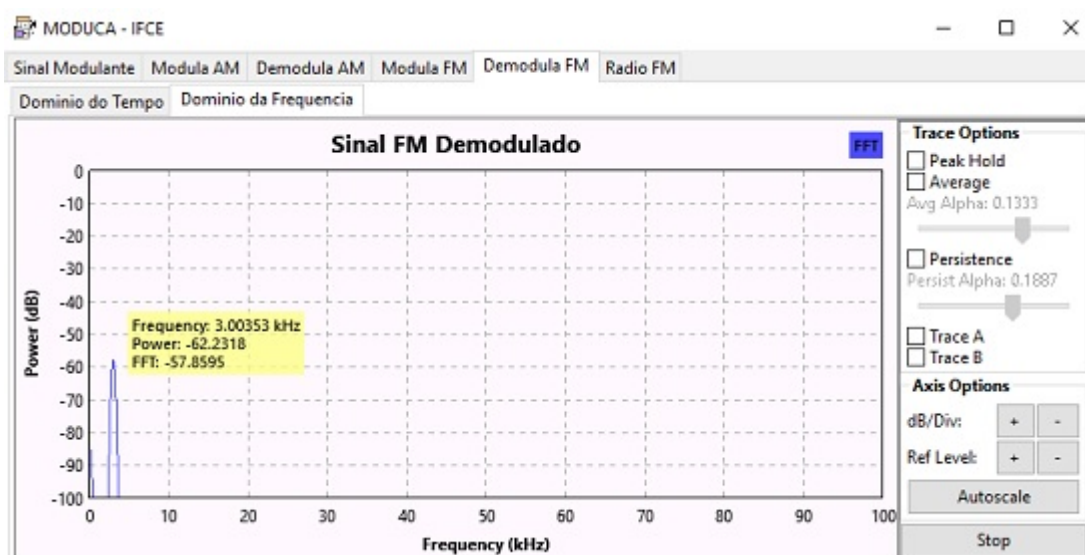
Figura 22 - Espectro do sinal da Figura 21 Fonte: O autor (2018)
