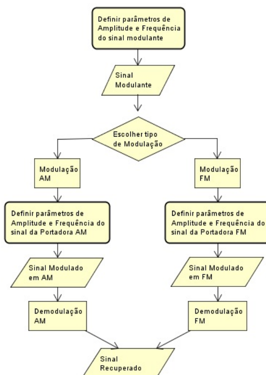
Figura 10 - Fluxograma do sistema MODUCA
