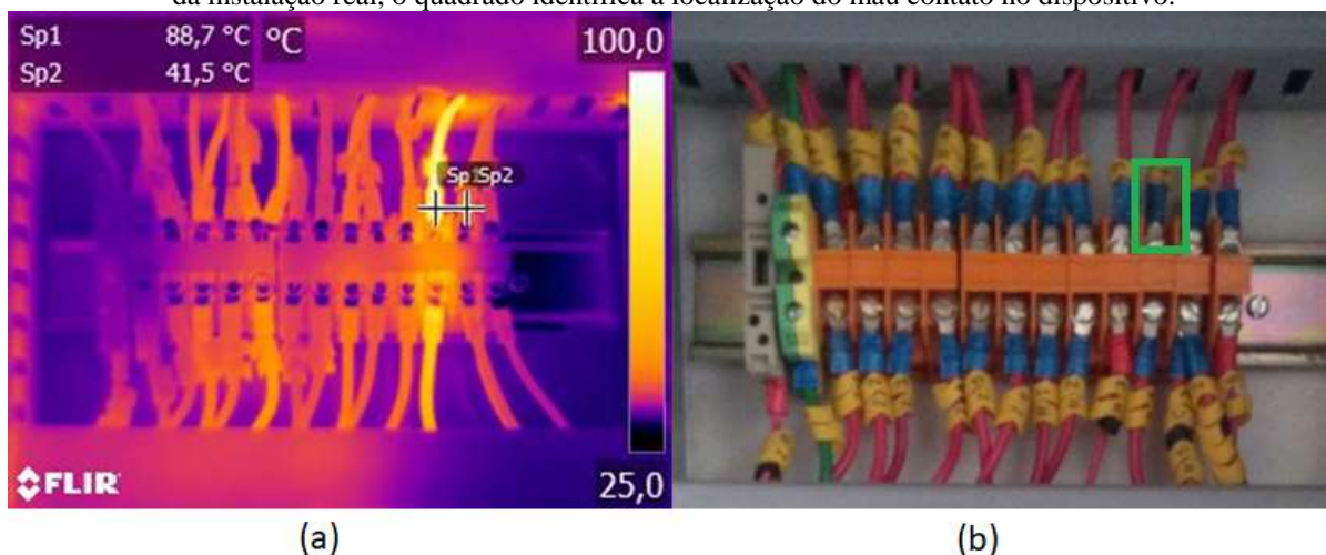
Figura 1 – (a) Termograma mostrando o mau contato inserido no condutor de alimentação da carga. (b) Imagem da instalação real, o quadrado identifica a localização do mau contato no dispositivo.
