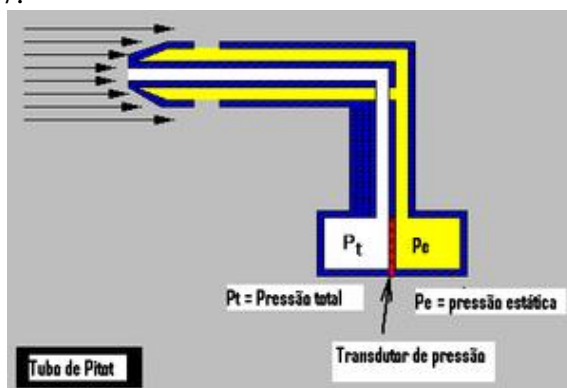
Figura 2 – Tubo de Pitot Fonte: COMMONSWIKI, 2007.
