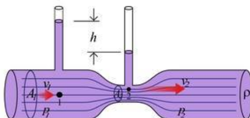
Figura 4 – Tubo de Venturi. Fonte: RODRIGUEZ.
