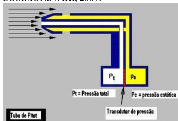
Figura 2 – Tubo de Pitot Fonte: COMMONSWIKI, 2007.
