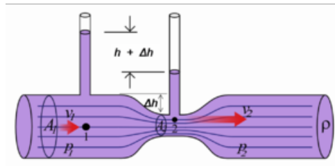
Figura 4 – Tubo de Venturi. Fonte: WIKIPÉDIA, 2006.
