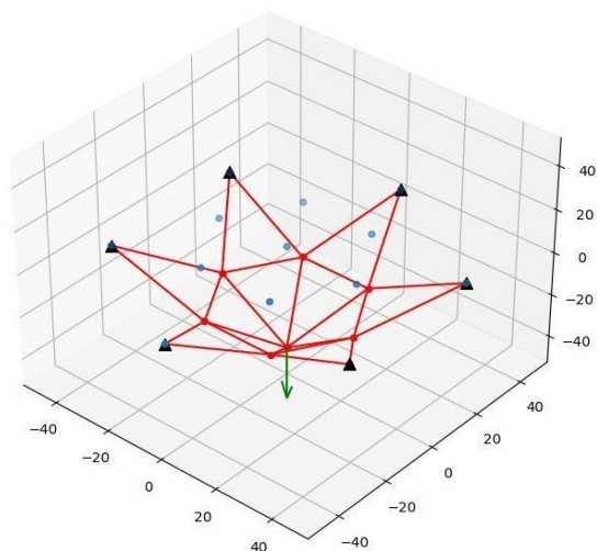
Figura 4 – Geometria deformada final do domo treliçado em formato de estrela.
