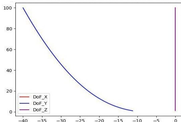
Figura 3 – Gráfico de resultado da força versus posições nodais vertical no nó central.
