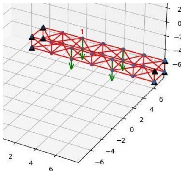
Figura 5 – Geometria inicial da viga treliçada.
