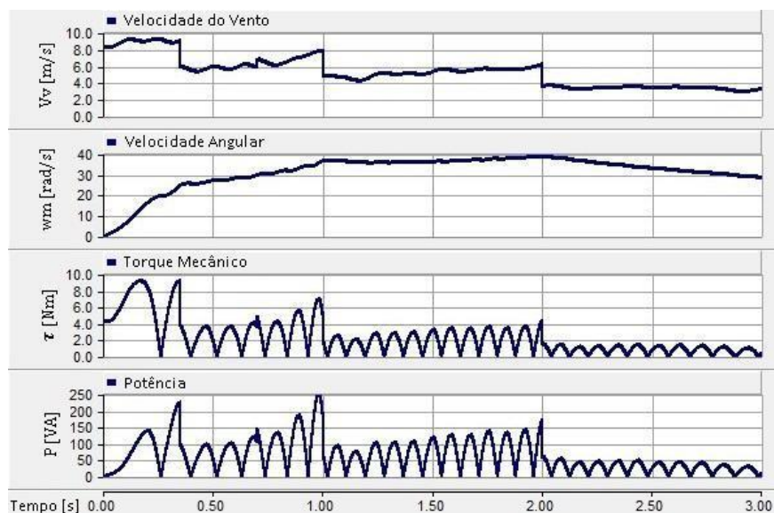
Figura 14 – Comportamento da turbina mediante a variação da velocidade do vento
