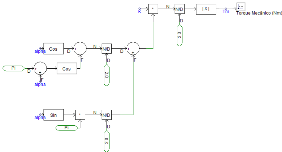
Figura 8 – Modelagem do Torque
