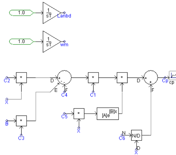
Figura 6 – Cálculo do coeficiente de potência da turbina
