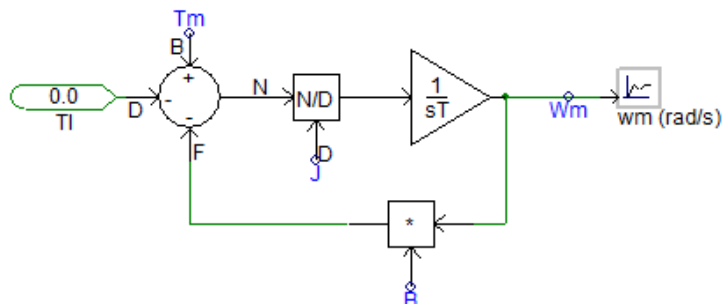
Figura 9 – Diagrama que calcula a velocidade angular da turbina
