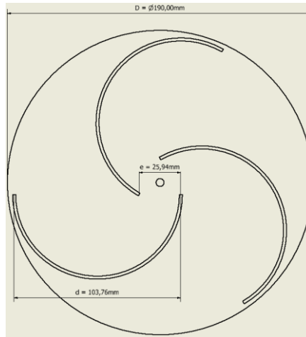
Figura 3 – Dimensionamento de um rotor Savonius
