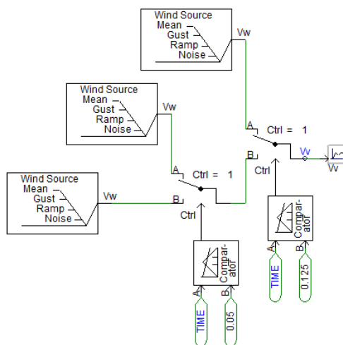
Figura 10 – Simulação da velocidade do vento
