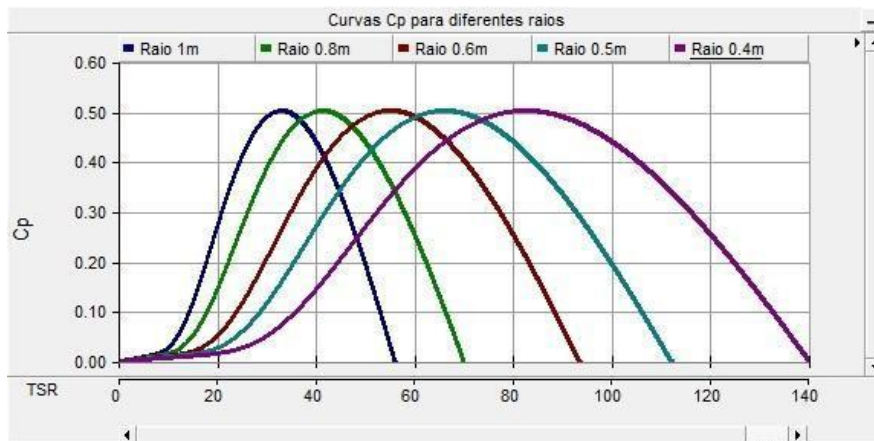
Figura 7 – Curvas de potências de rotor Savonius com vários raios
