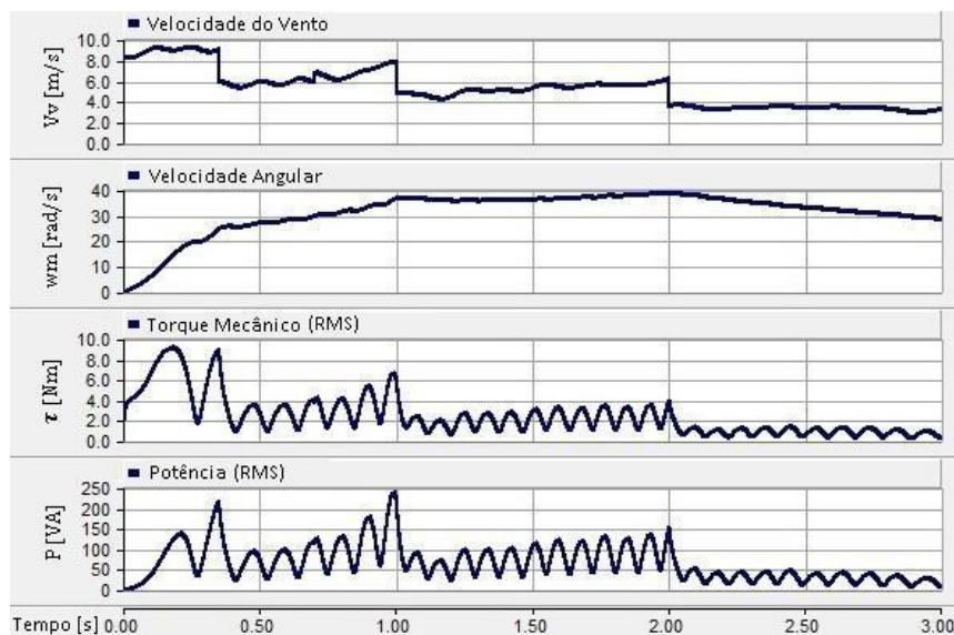
Figura 15 – Comportamento da turbina com valores RMS
