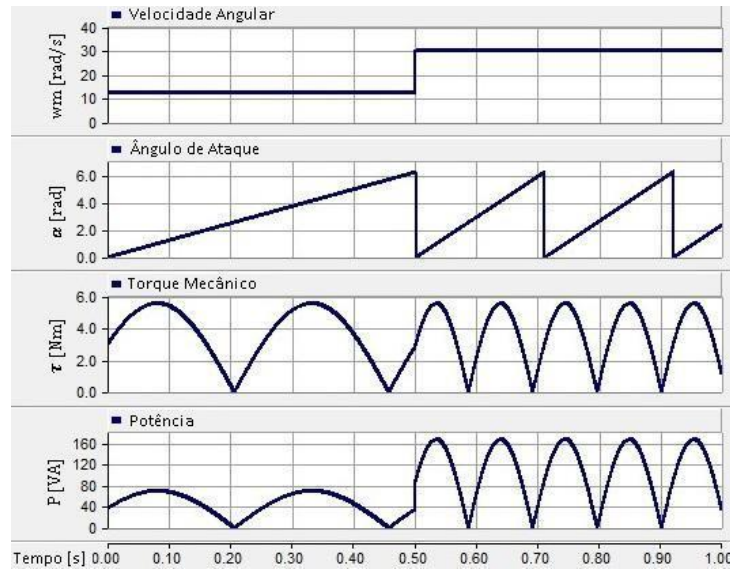
Figura 13 – Comportamento da turbina sob variação da velocidade angular
