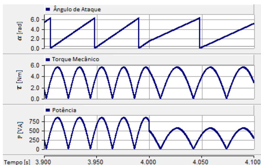
Figura 12 – Comportamento da turbina sob variação da velocidade angular
