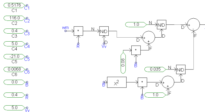
Figura 5 – Diagrama do cálculo de \lambda
