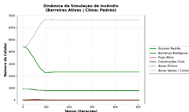
Figura 4 – Gráfico de evolução espaço-temporal e dinâmica populacional da simulação estocástica de incêndio florestal
