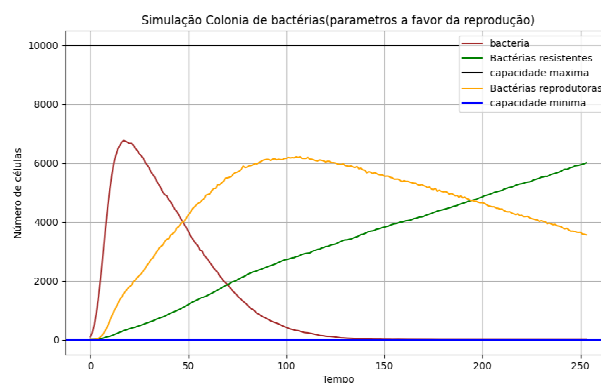
Figura 6 – Gráfico de análise visual e quantitativa da competição espacial em colônias bacterianas parametrizadas a favor da reprodução.
