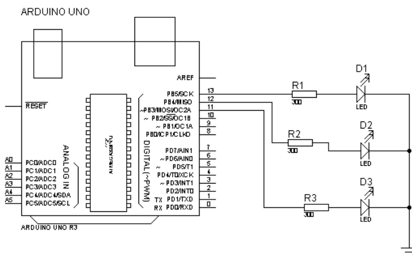
Figura 4: Circuito eletrônico para o acionamento dos LED's.
