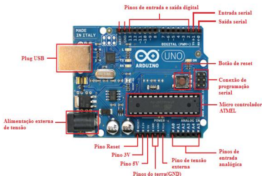
Figura 1: Arduino UNO
