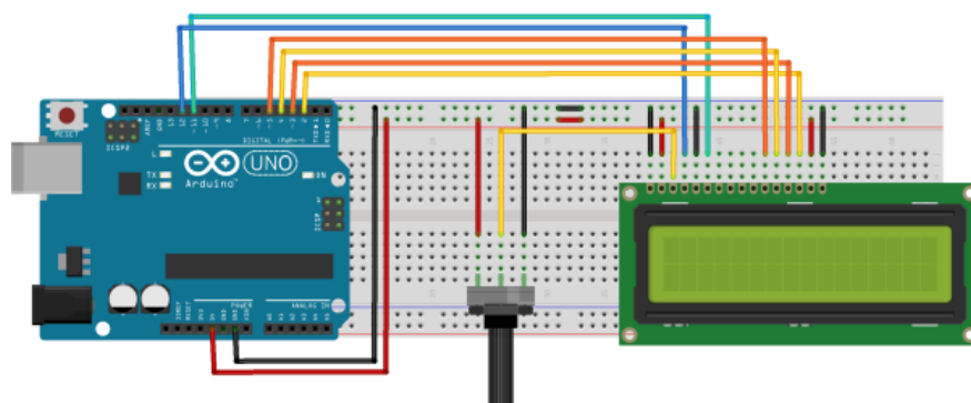
Figura 5: Esquemático proposto na aula
