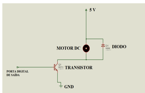
Figura 7: Circuito proposto
